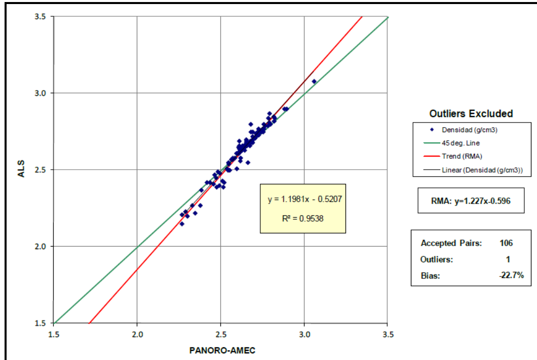
Figure 11.1 Panoro Unsealed versus ALS Chemex Wax Sealed Dry In Situ Bulk Density
